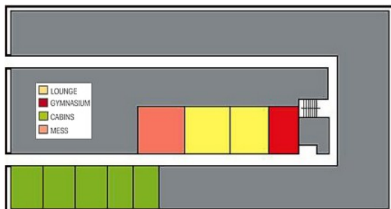
Plan des 11. Decks
