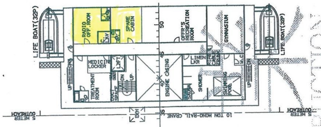
Deckplan des F-Deck
