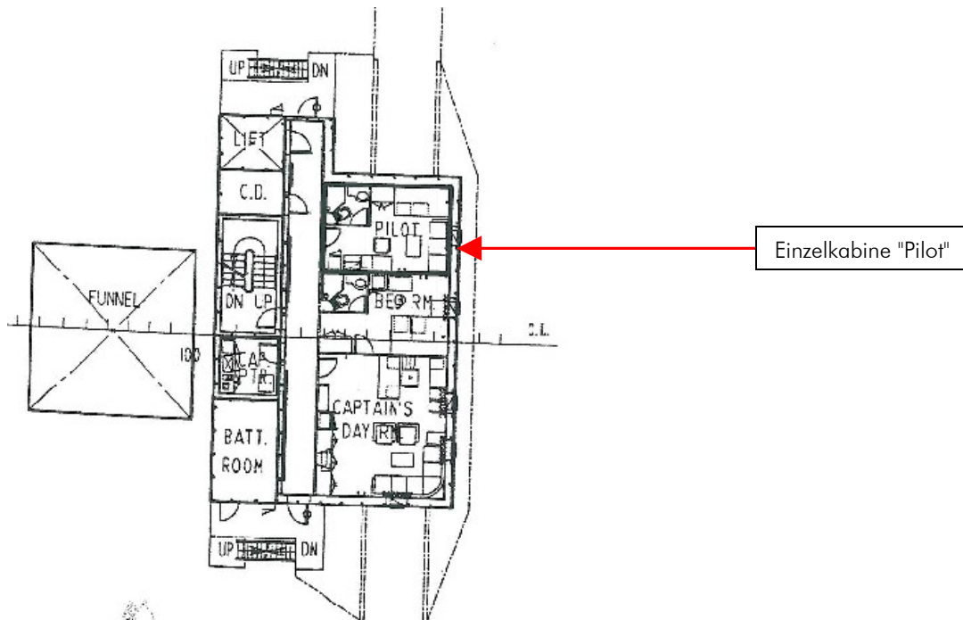
Deckplan des F-Deck mit der Einzelkabine "Pilot"
