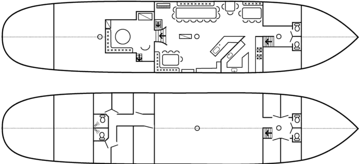
Deckplan der Oosterschelde
