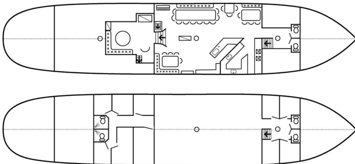
Deckplan der Oosterschelde
