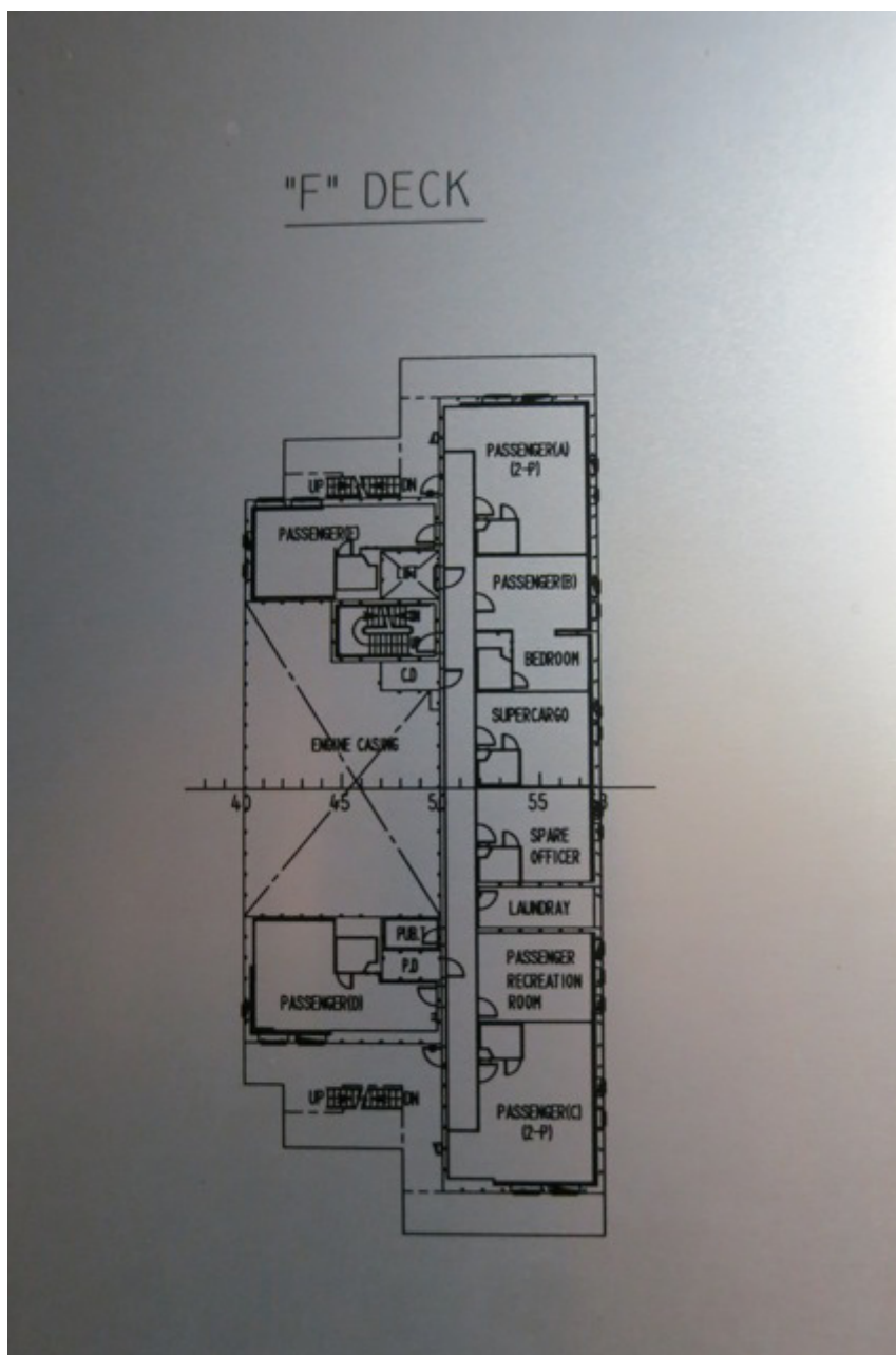
Deckplan des Passagierdecks
